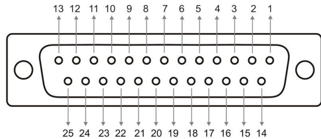
TECO-JSDE (DB25F)
