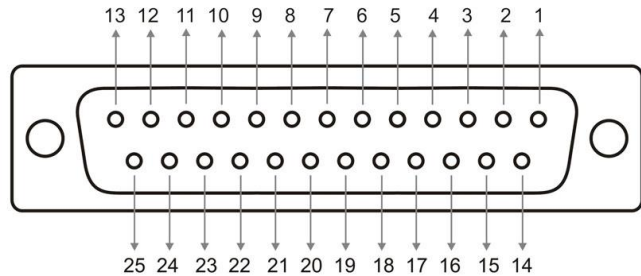
TETA D2 (DB25)
