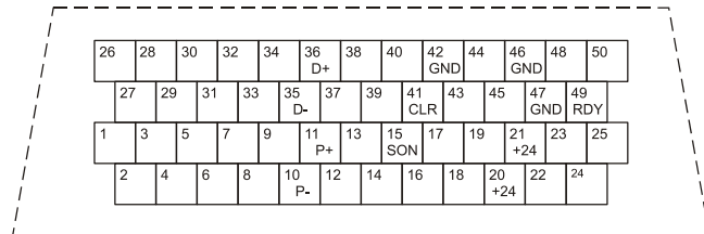
MR-JE (50 Pins)
