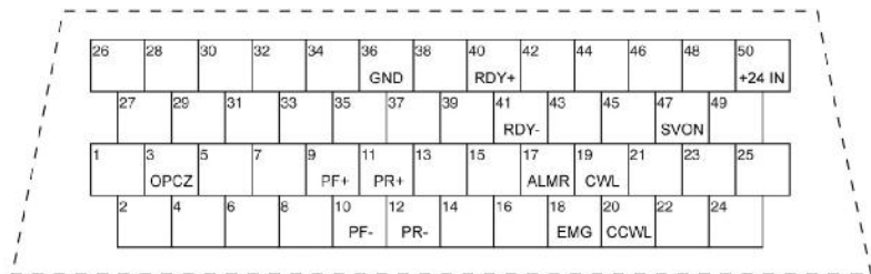
APD-VS (50 Pins)
