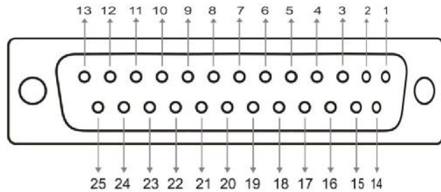
ASDA-B (DB25F)
