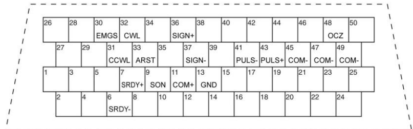
ASDA-A2 (50 Pins)
