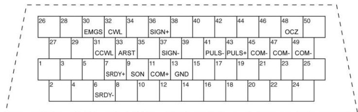
ASDA-A2 (DB25F)
