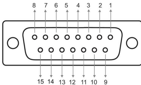
PC-Pro 8A (DB15F)
